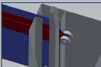
Winddrucksicherung
